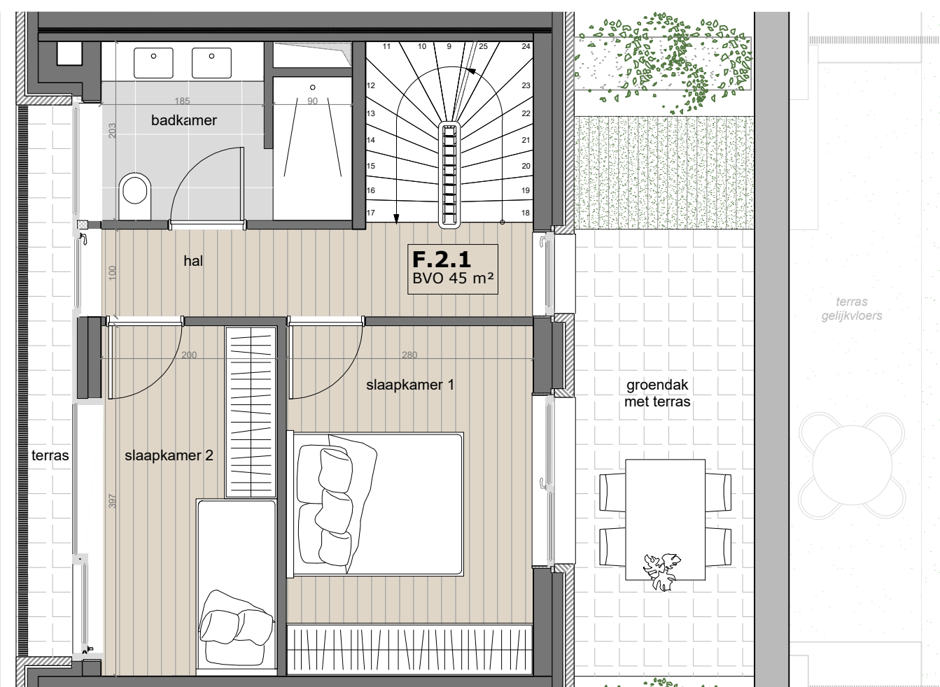
EERSTE VERDIEP
